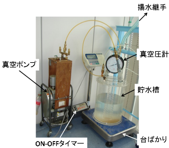
真空ポンプ(電動機出力:200 W, 排気速度:50 L/min)
