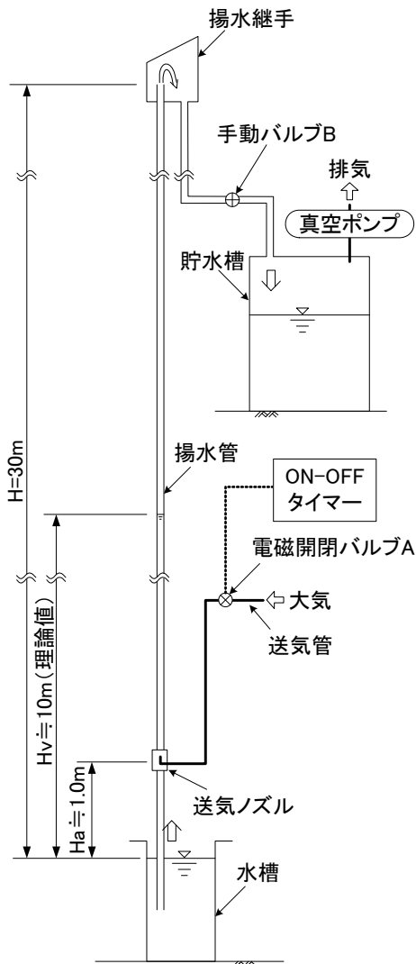
真空ポンプ揚水実験装置の概要
