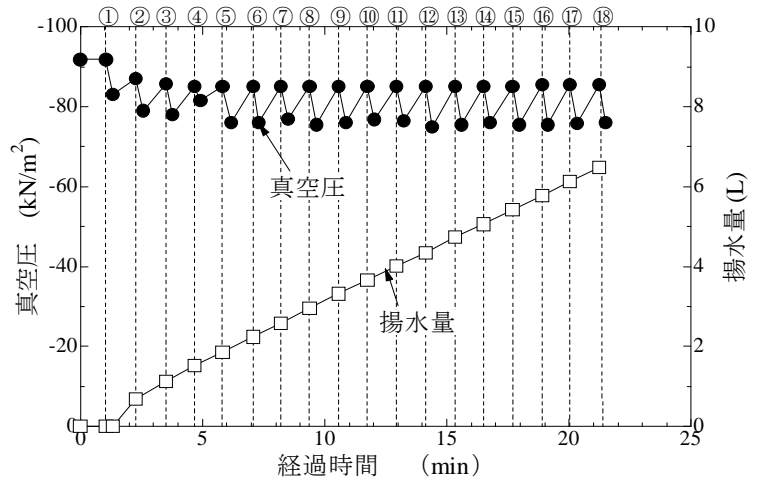
真空圧と揚水量の経時変化の一例
